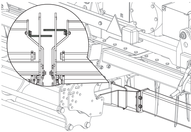
FIG. 12 MekFold 180
