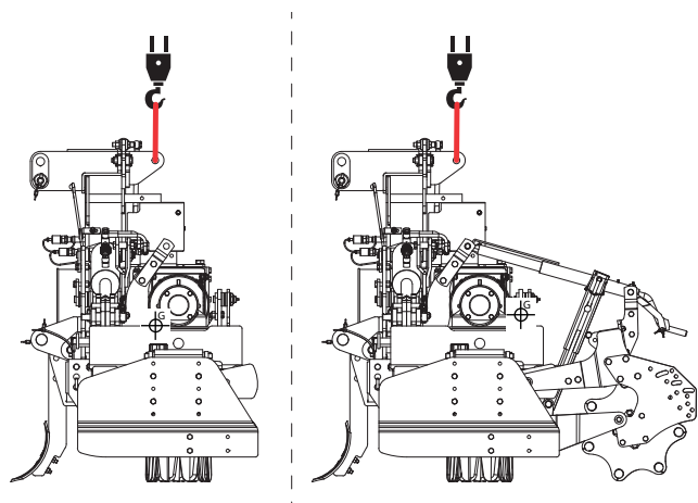
FIG. 5 Maschinenbewegung
