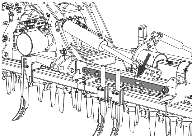
FIG. 35 Sicherheitsstange auf dem Gestell
